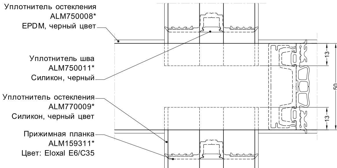
Стык профилей. Вид с фасада.
