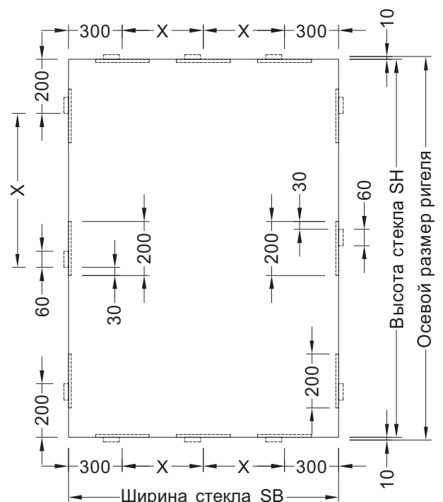
Схема остекления
