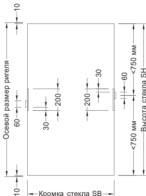
Схема остекления
